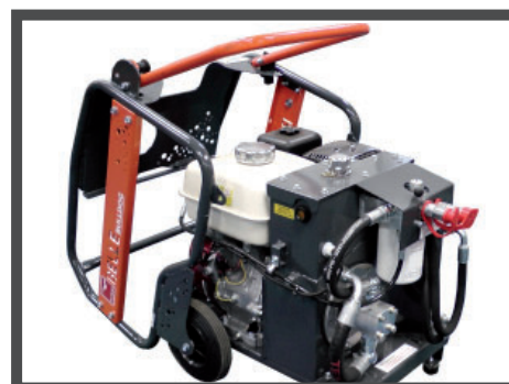
Telaio inclinabile per agevolare interventi di manutenzione
